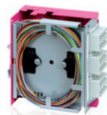
Spleißkassette
