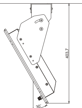
STAND ANGLE
